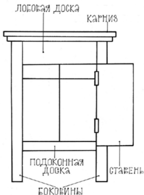
Рис. 1 Элементы наличника
